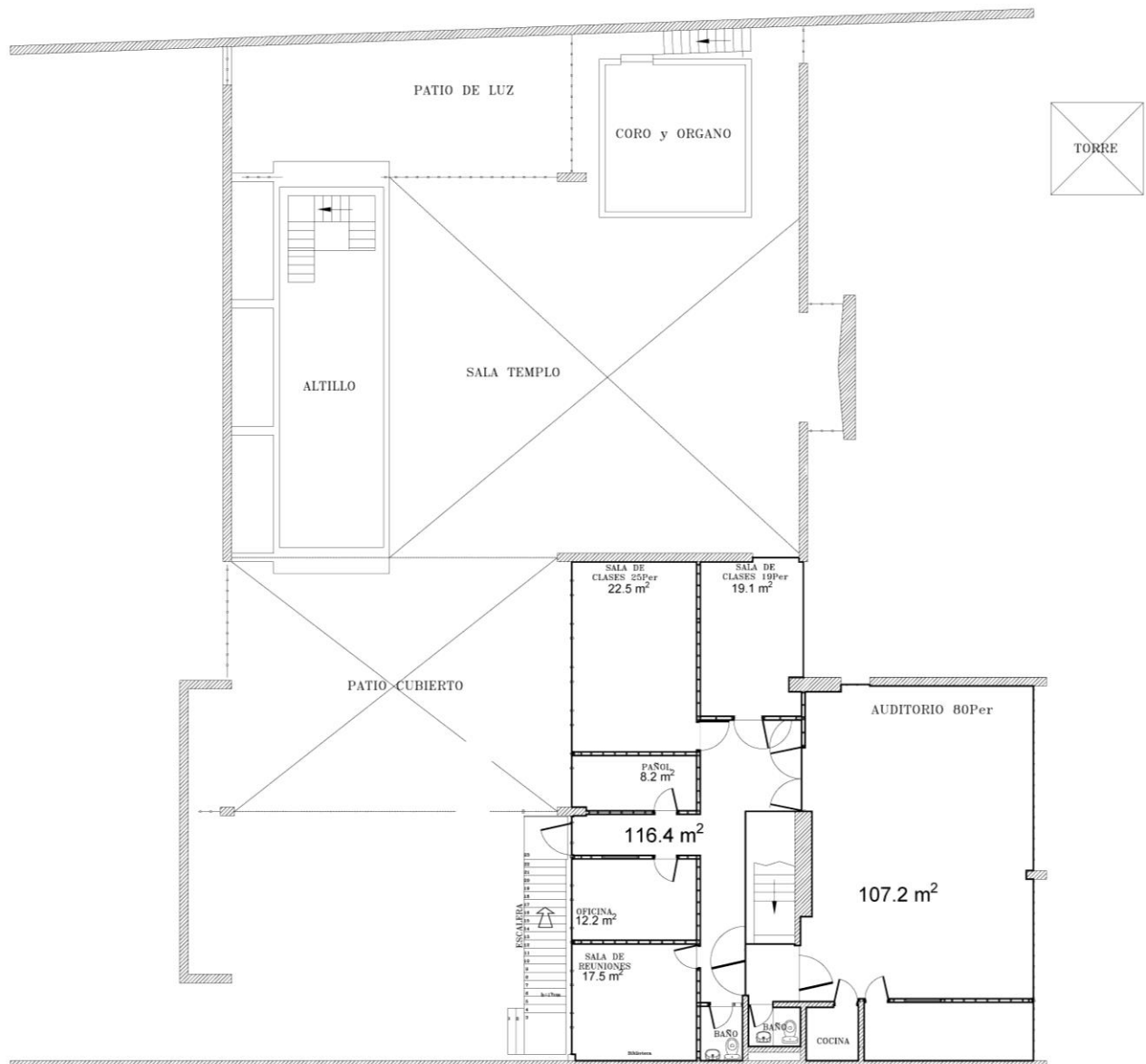
Planta de arquitectura del segundo piso
