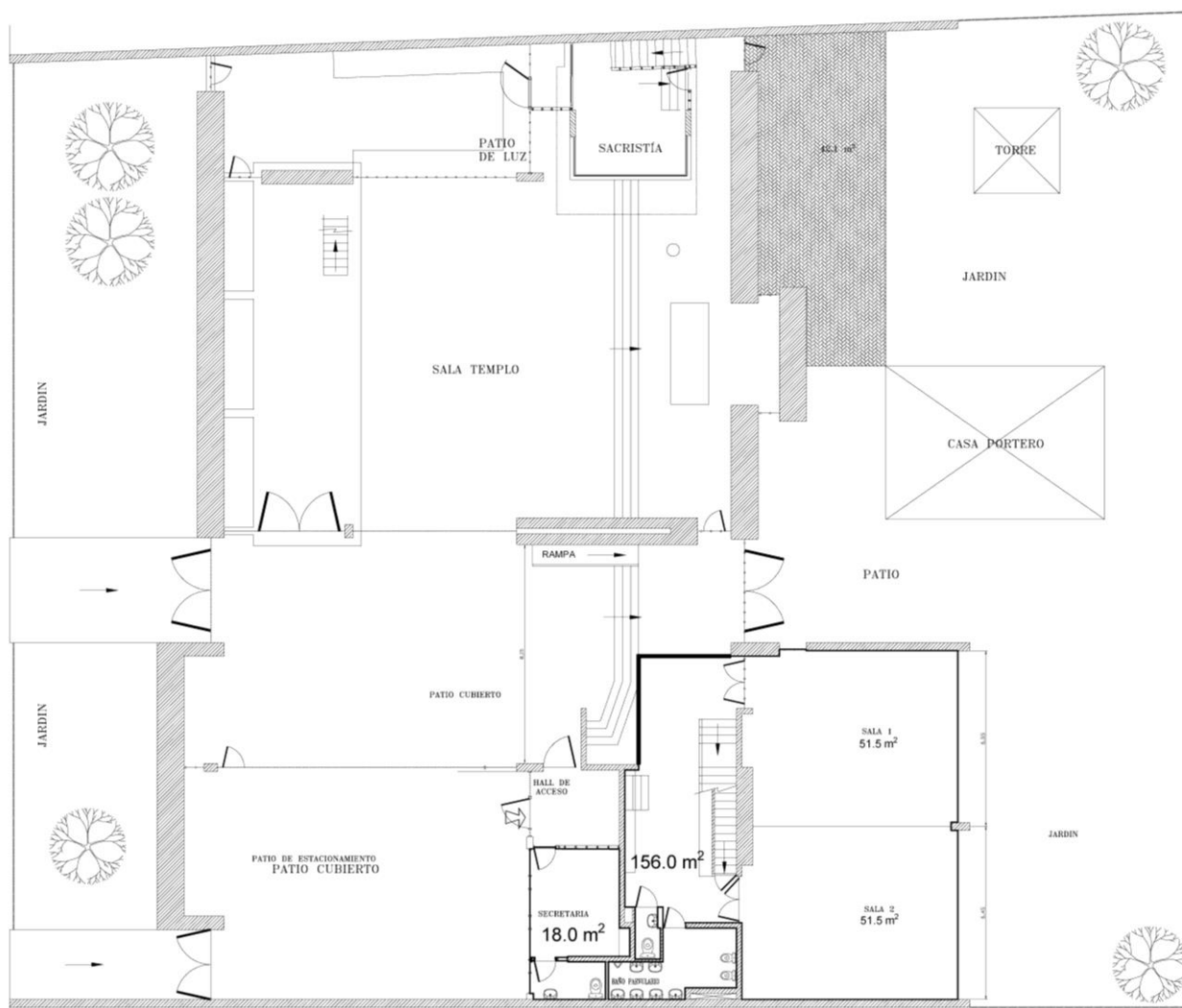
Planta de arquitectura del primer piso y terreno
